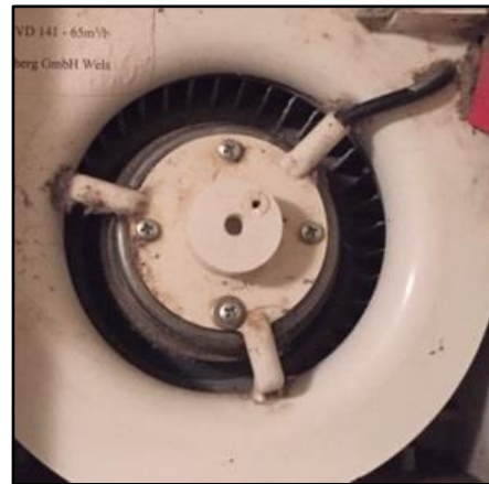
Abb. 1.: Motortrageplatte in gutem Zustand
